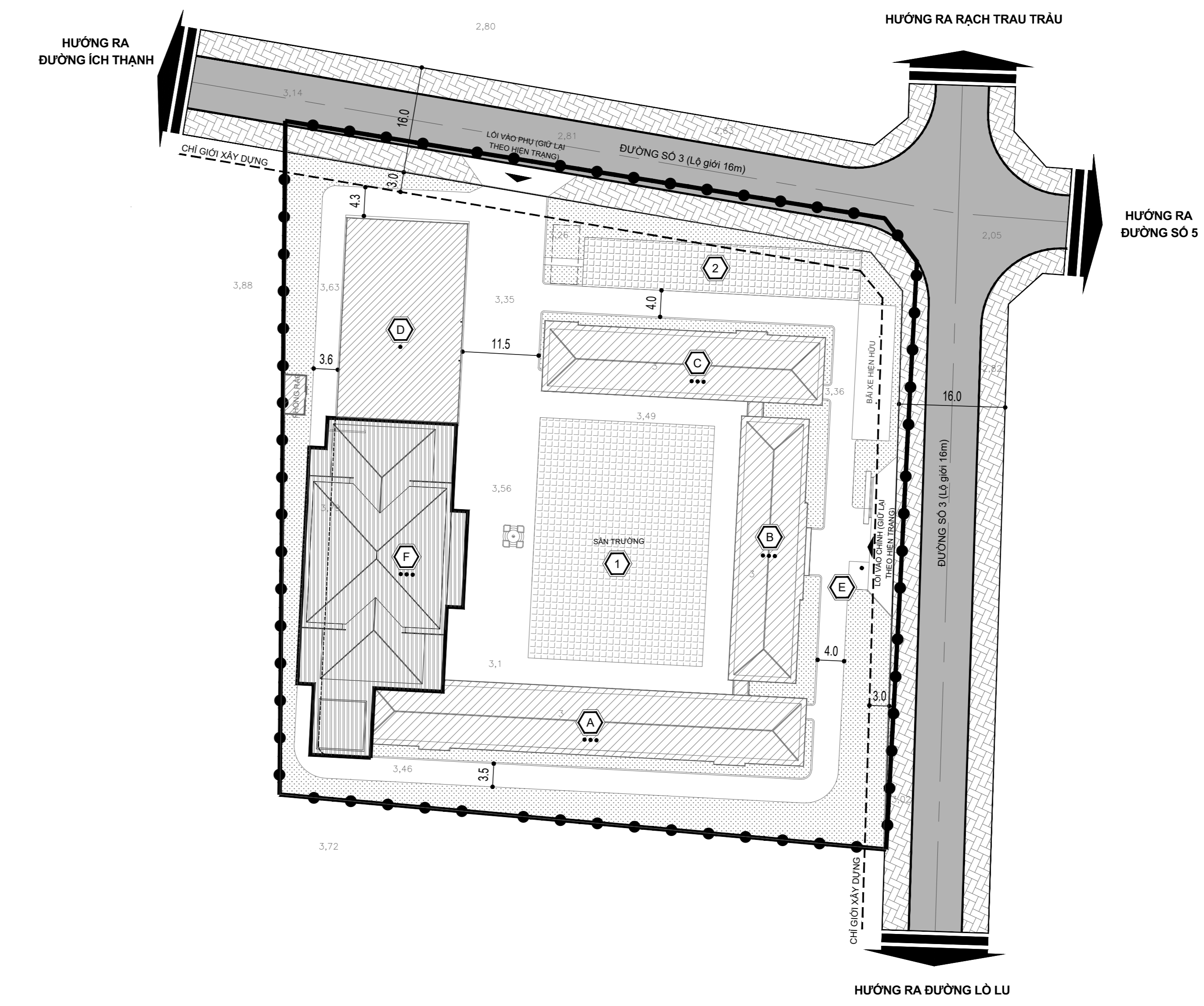
BẢN VẼ TỔNG MẶT BẰNG - TỶ LỆ 1/500
